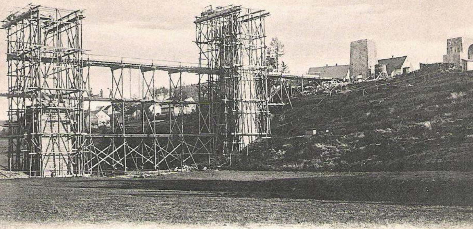
Die im Bau befindliche Eisenbahnbrücke bei Franzthal, der Linie Nixdorf-Sebnitz (Totale Länge 190,0 m, 5 Felder à 38 m, 4 Pfeiler von 12–29 m Höhe. Grösste Höhe der Fahrbahn 34 m)
